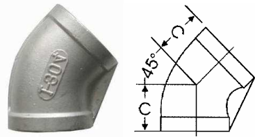
45° 弯头 45° ELBOW FIG NO.5
