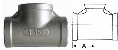
三通 TEE FIG NO.2
