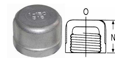
圆管帽 CAP FIG NO.12
