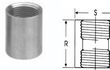
光面接头 COUPLING FIG NO.15
