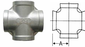
四通 CROSS FIG NO.3
